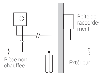
Toujours placer la sonde à l'endroit le plus froid de l'installation
