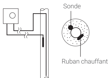
Fixer la sonde à la tuyauterie (par ex. avec du ruban adhésif en aluminium)
